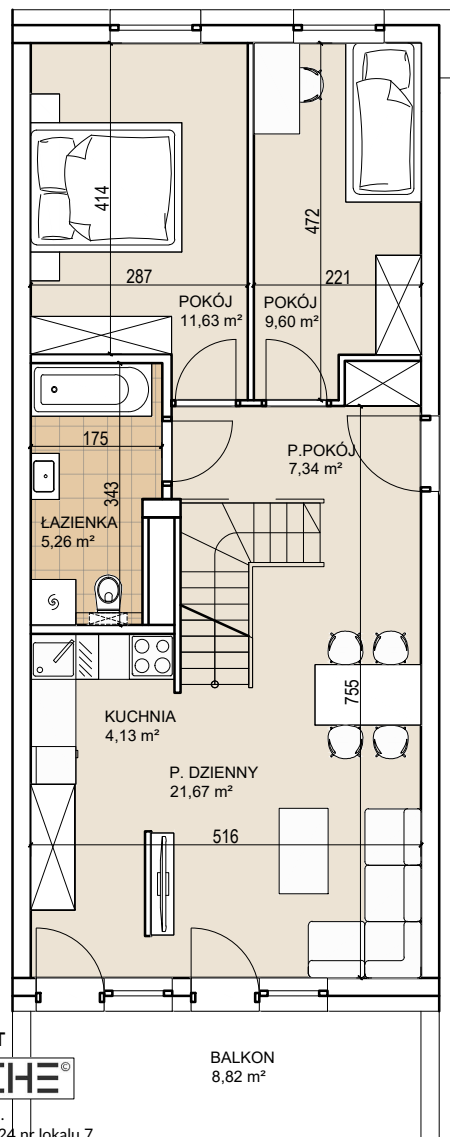
Poziom 1
