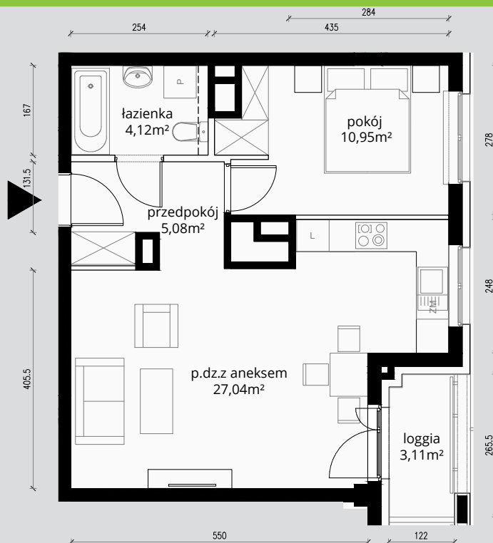
RZUT KONDYGNACJI 10 PIĘTRO
