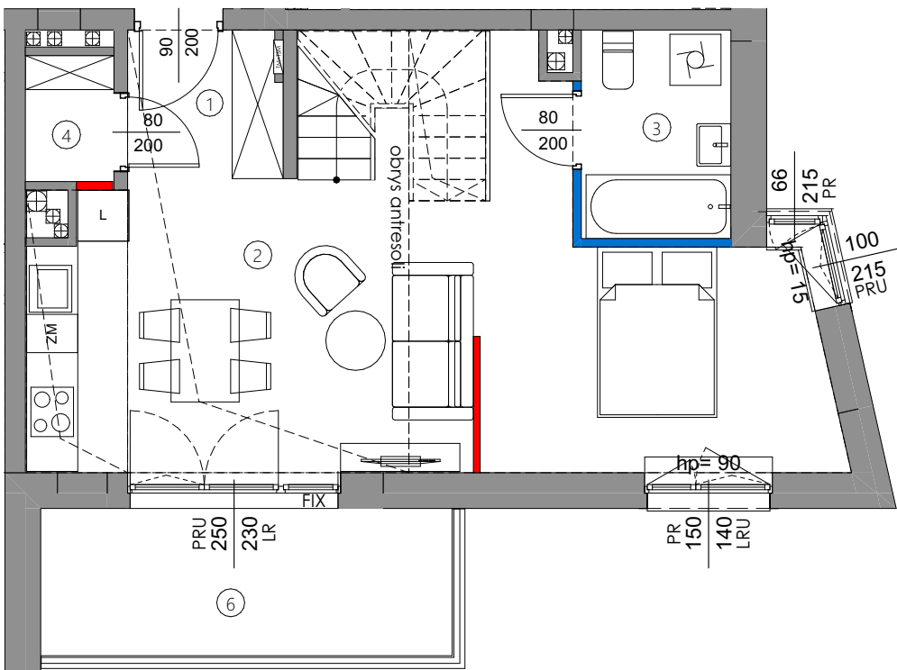
POZIOM DOLNY
