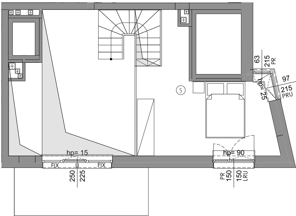
POZIOM ANTRESOLI
