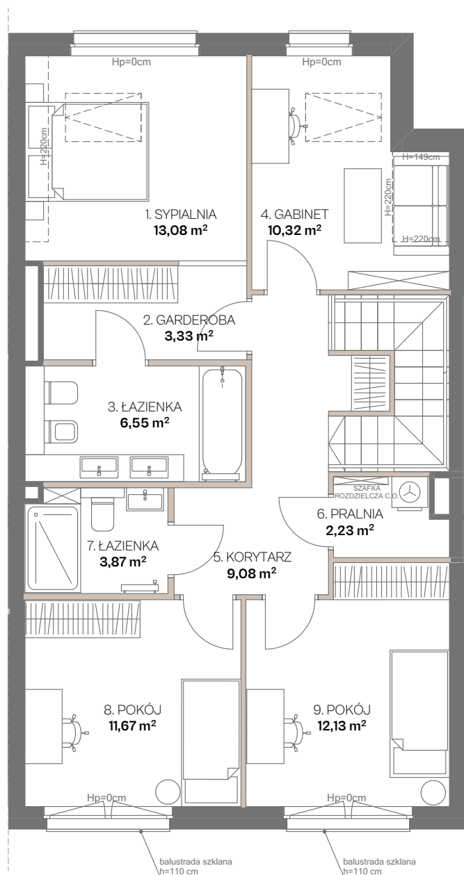
RZUT 1. PIĘTRA
