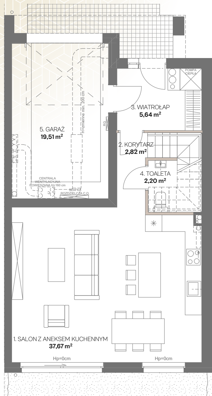
RZUT PARTERU
