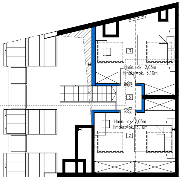
POZIOM + I
