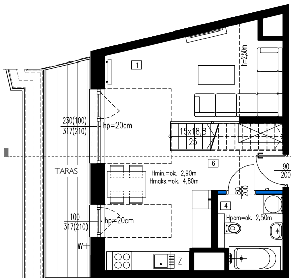
POZIOM 0
