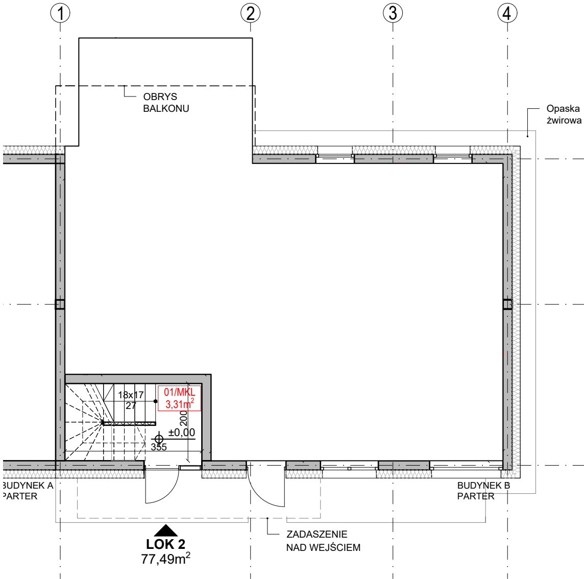
RZUT PARTERU
