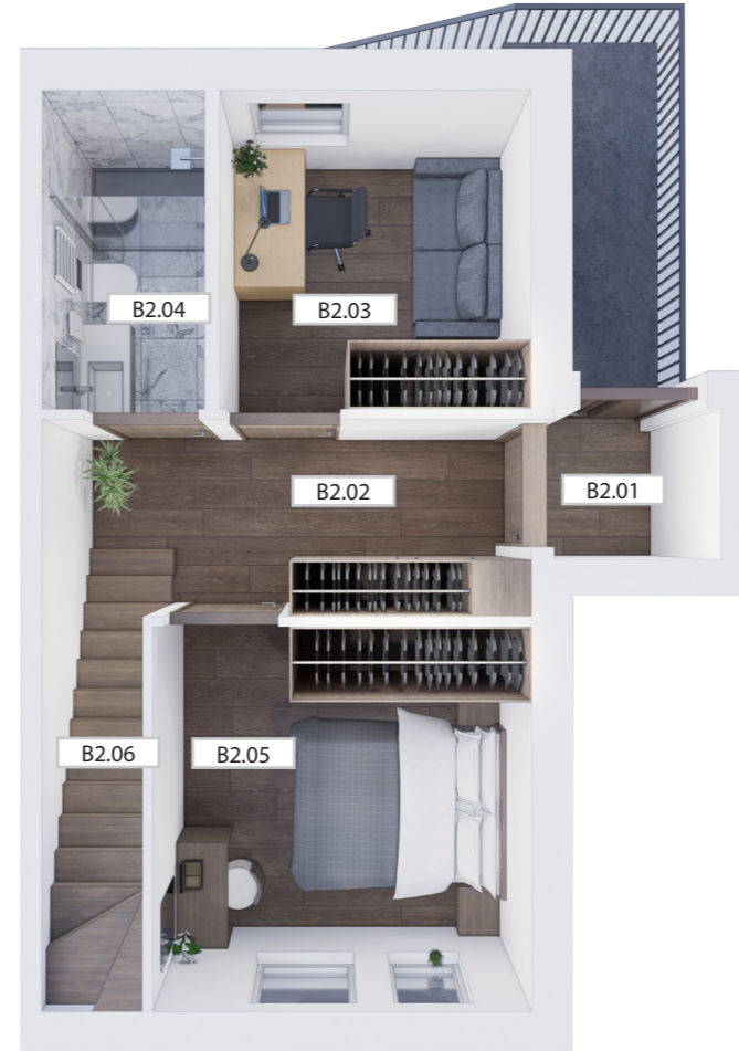
RZUT PIĘTRA 1
