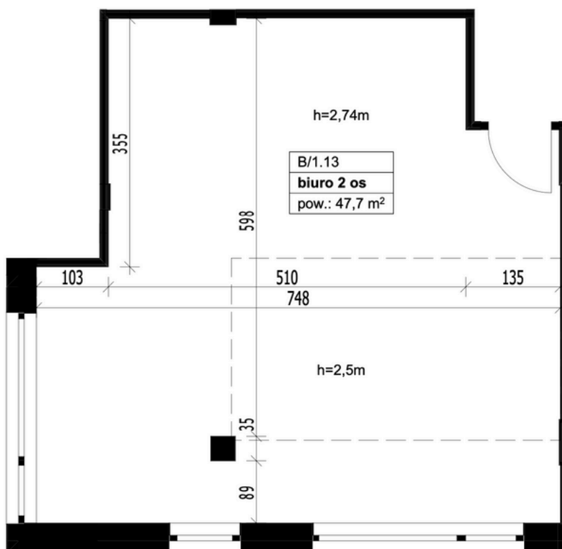
KONDYGNACJA: 1 PIĘTRO
