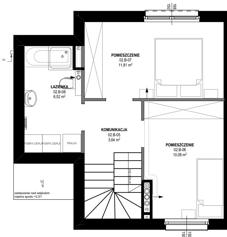
RZUT 2 PIĘTRA
