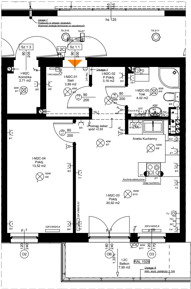
RZUT w skali 1:100
