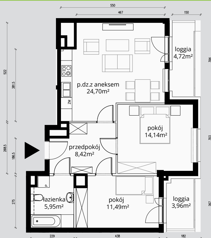
RZUT KONDYGNACJI 17 PIĘTRO
