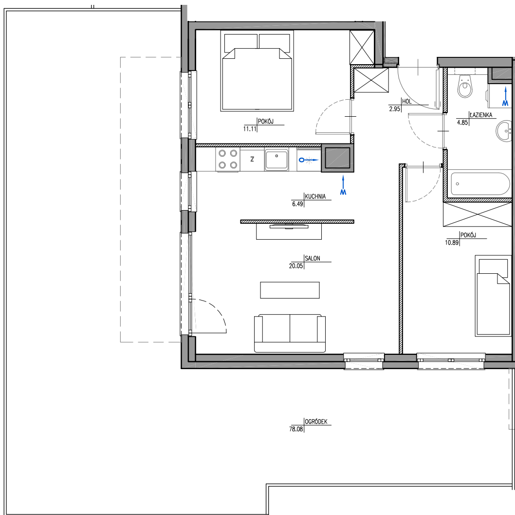
SCHEMAT LOKALU MIESZKALNEGO NA RZUCIE
