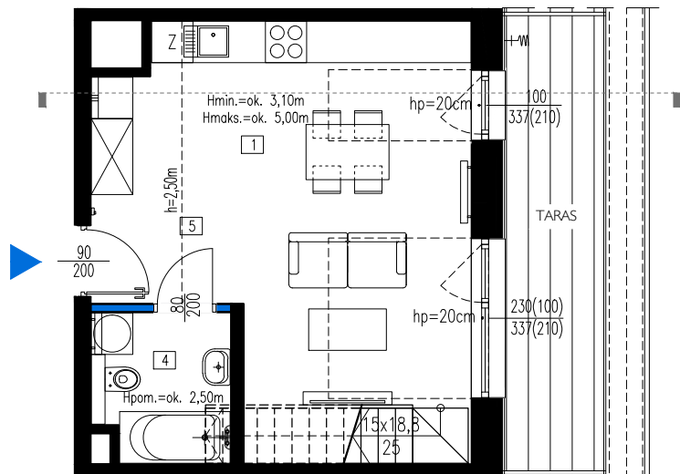
POZIOM 0
