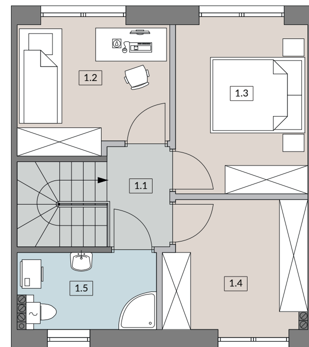
RZUT PIĘTRA
