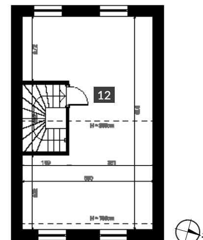
Rzut poddasza
