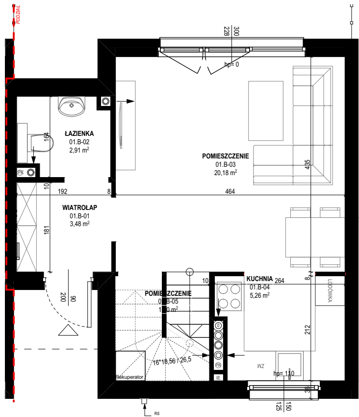
RZUT PARTERU
