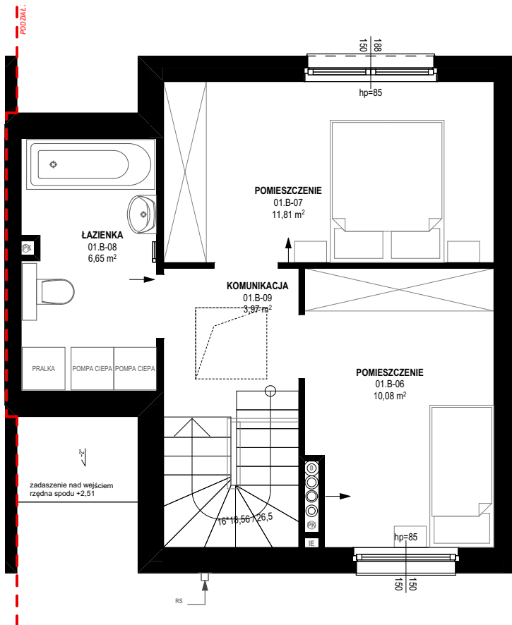
RZUT 1 PIĘTRA
