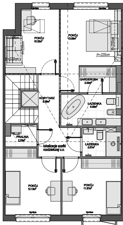
PIĘTRO
