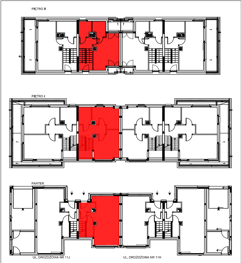
SCHEMAT KONDYGNACJI BUDYNKU NR 11H, 11J.
