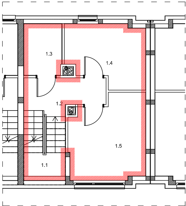
RZUTPIĘTRA I-GO BUDYNKU NR 11J LOKAL MIESZKALNY NR 1
