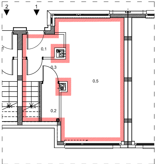
RZUT PARTERU BUDYNKU NR 11J LOKAL MIESZKALNY NR 1
