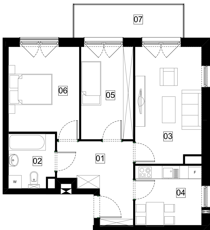
Wykaz pomieszczeń
