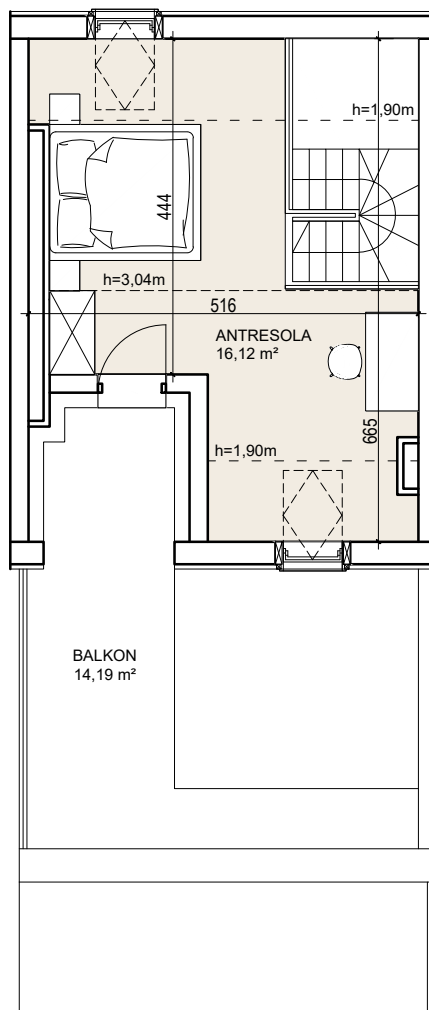
Poziom 2 (antresola)
