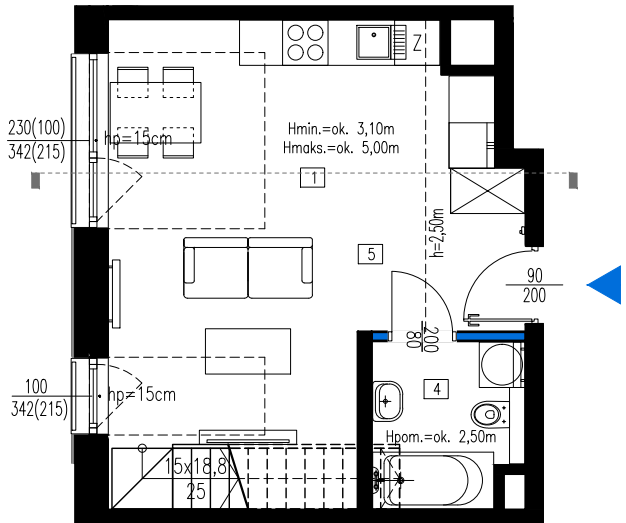
POZIOM 0
