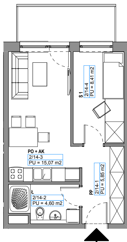
RZUT LOKALU 1 : 100
