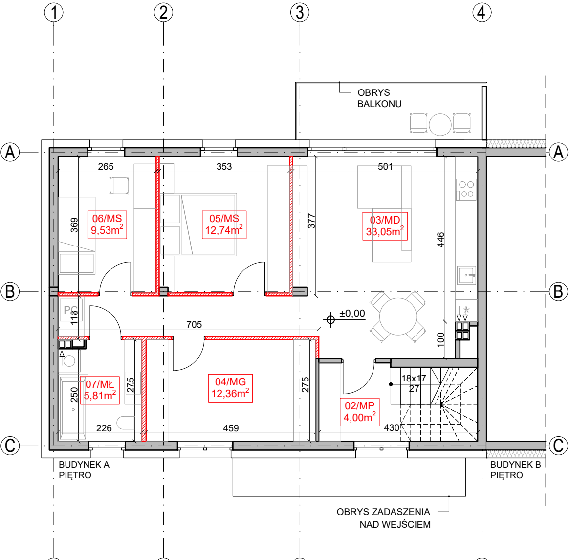
RZUT PIĘTRA
