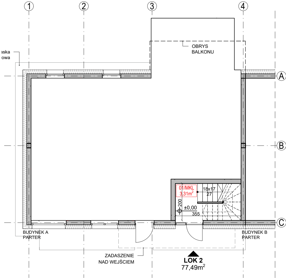
RZUT PARTERU
