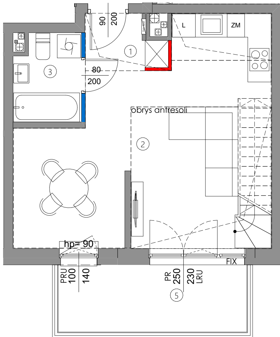
POZIOM DOLNY
