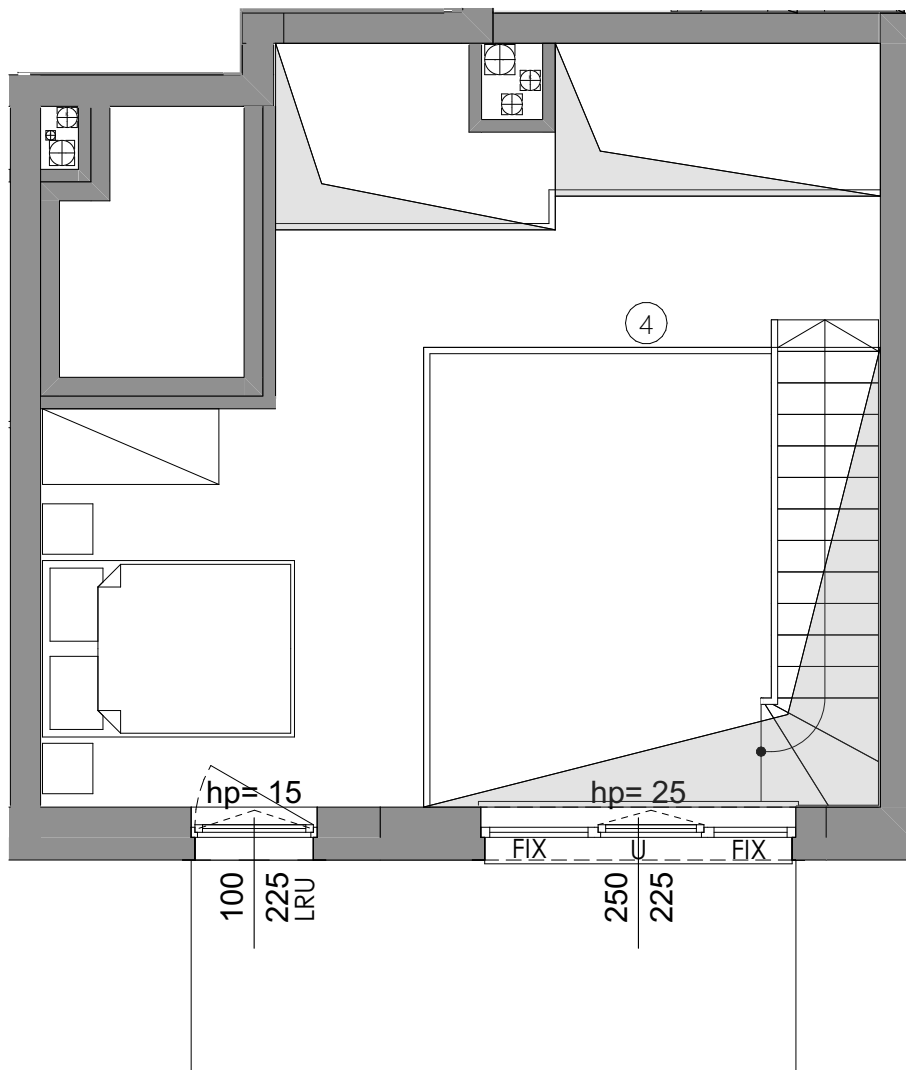
POZIOM ANTRESOLI
