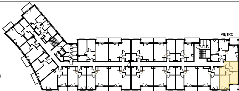
RZUT KONDYGNACJI
