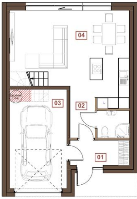
RZUT PARTERU
