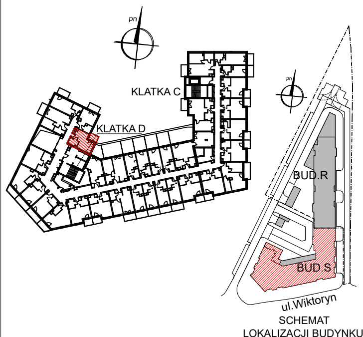
SCHEMAT MIKROAPARTAMENTU NA RZUCIE KONDYGNACJI
