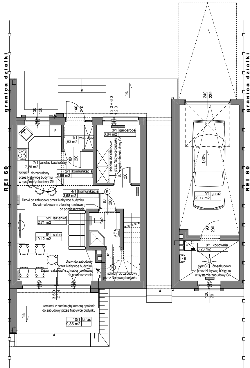
VILLA CAMPINA OŻARÓW MAZOWIECKI, SZEREG F06 - BUDYNEK ALICJA ŚRODKOWY, MODUŁY OD S129 DO S131
