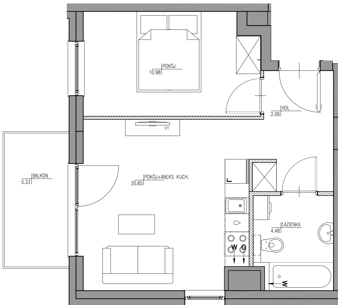
SCHEMAT LOKALU MIESZKALNEGO NA PIĘTRZE
