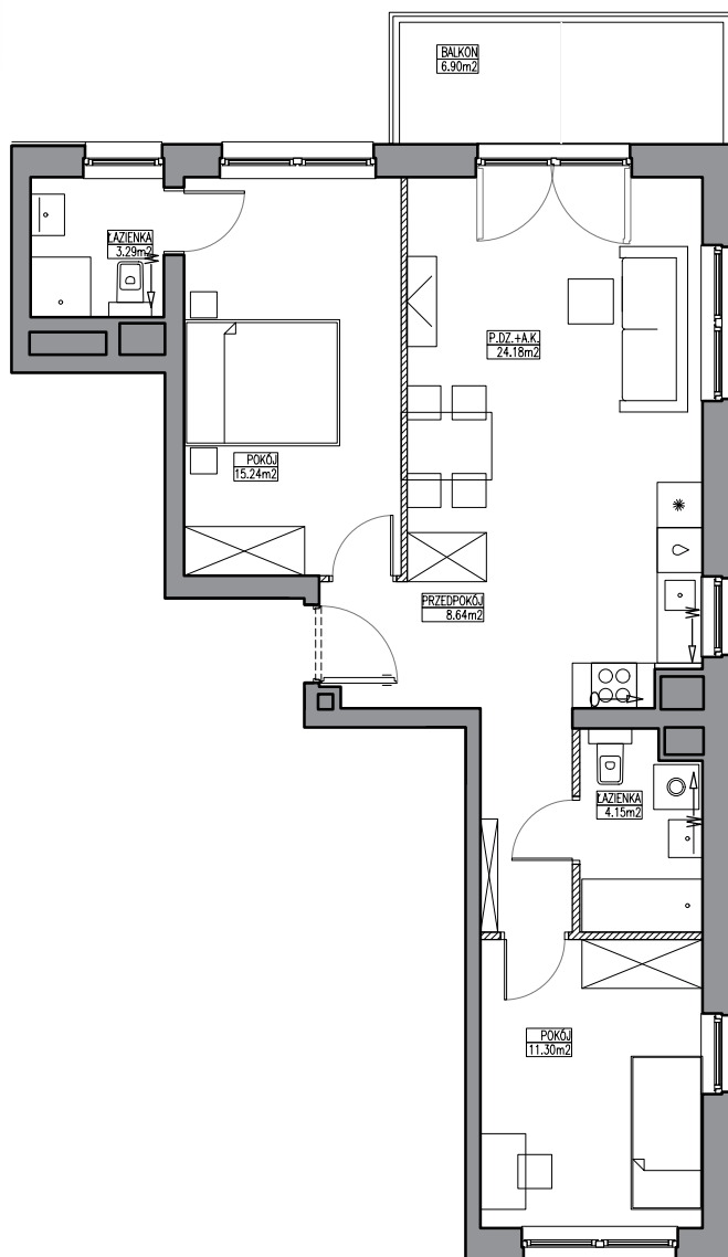
SCHEMAT LOKALU MIESZKALNEGO NA 4 PIĘTRZE
