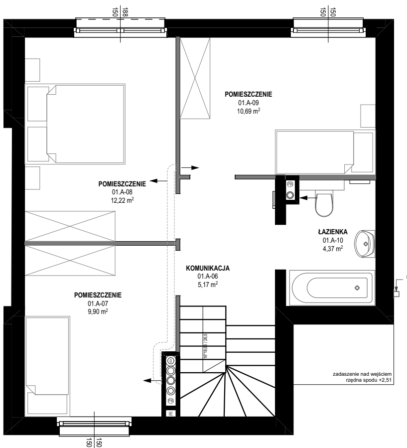
RZUT 1 PIĘTRA
