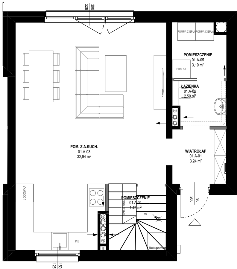
RZUT PARTERU
