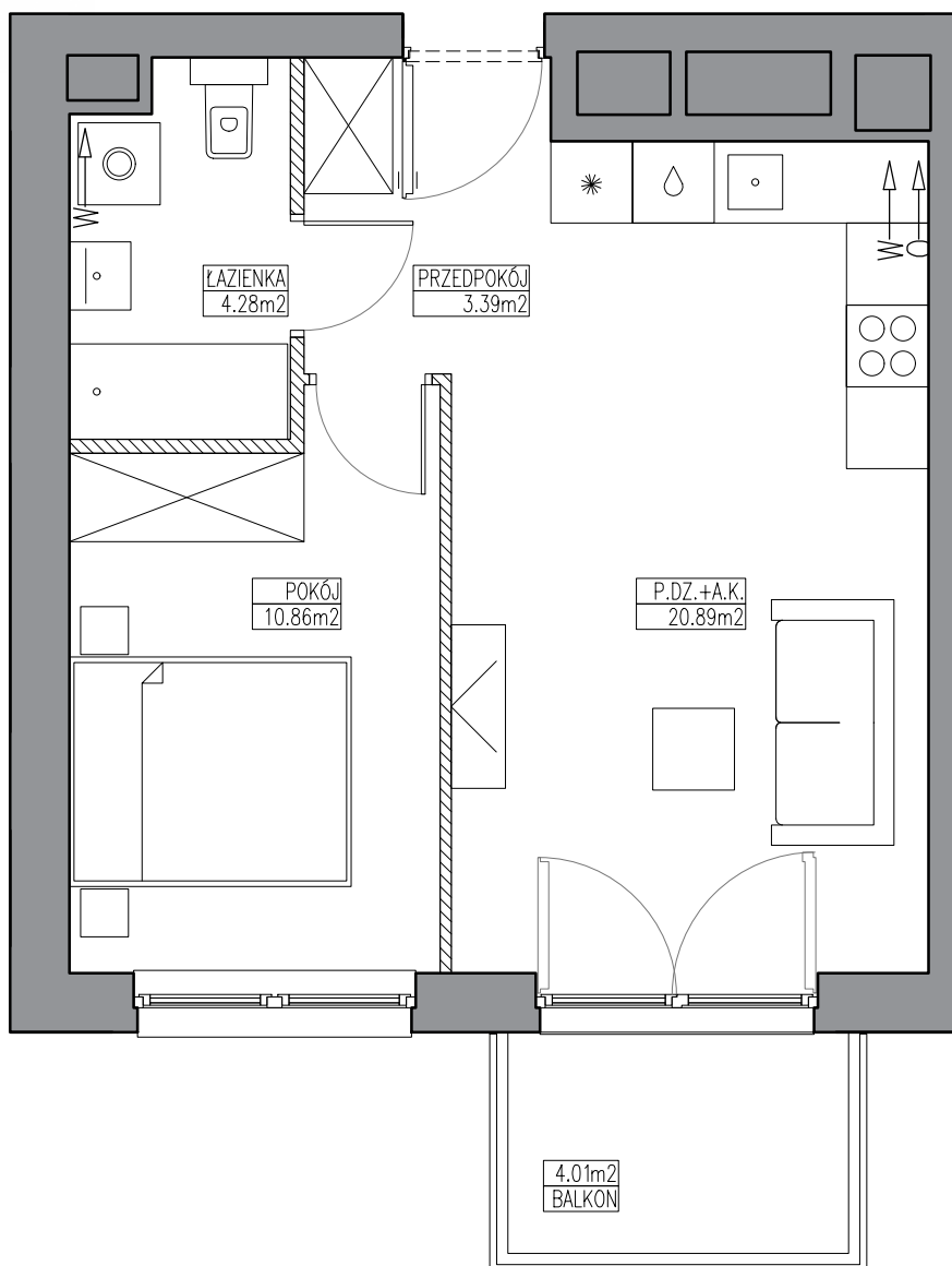
SCHEMAT LOKALU MIESZKALNEGO NA 1 PIĘTRZE
