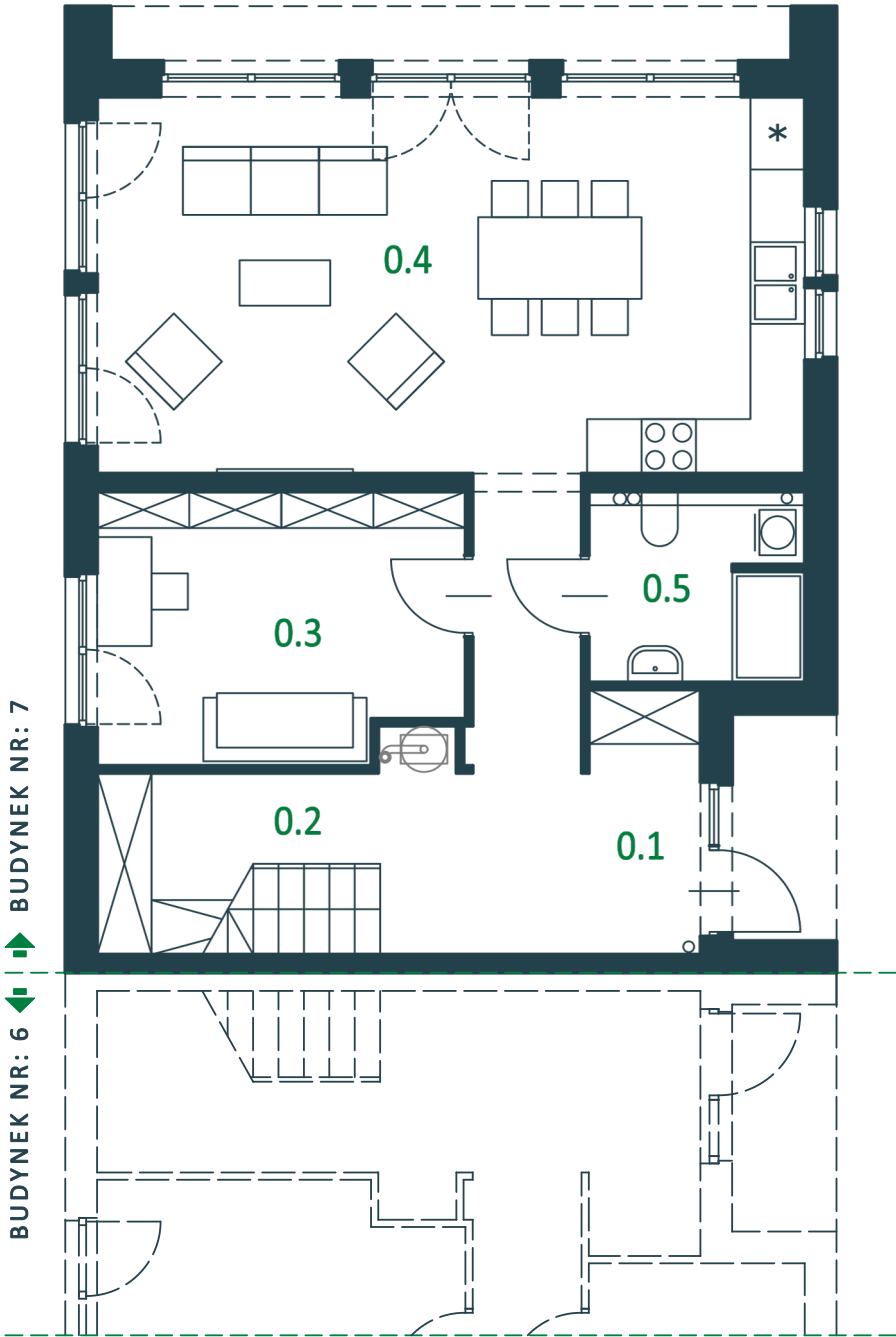
RZUT PARTERU
