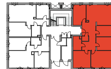
Schemat kondygnacji
