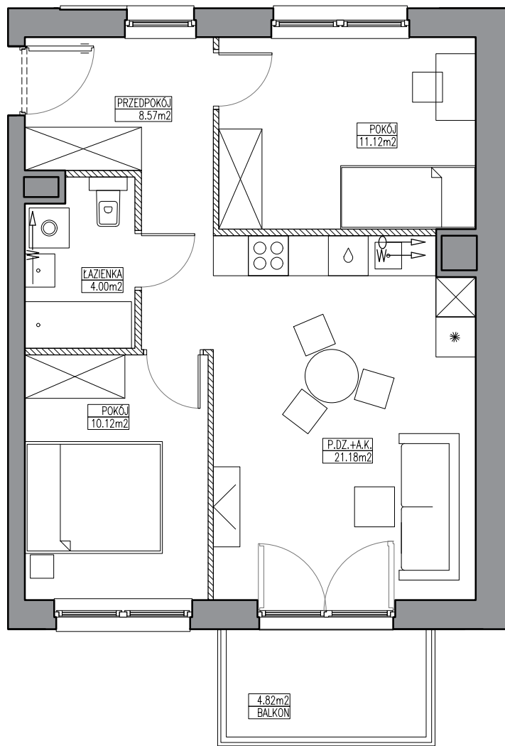
SCHEMAT LOKALU MIESZKALNEGO NA 2 PIĘTRZE
