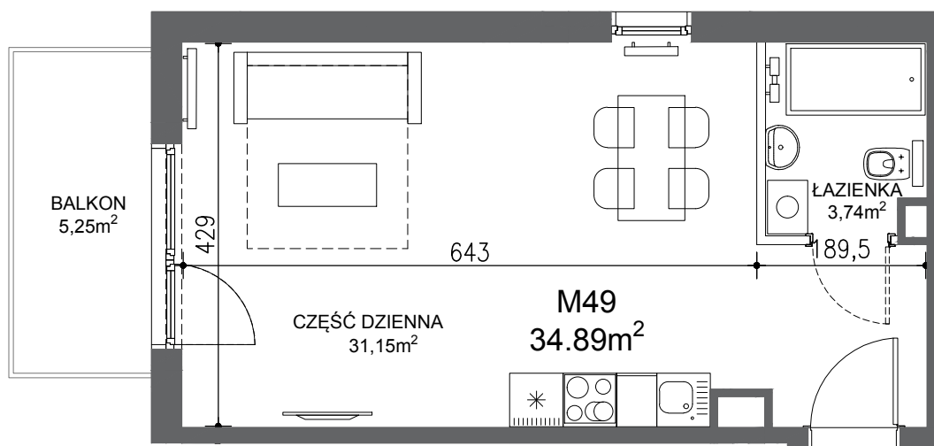
RZUT MIESZKANIA
