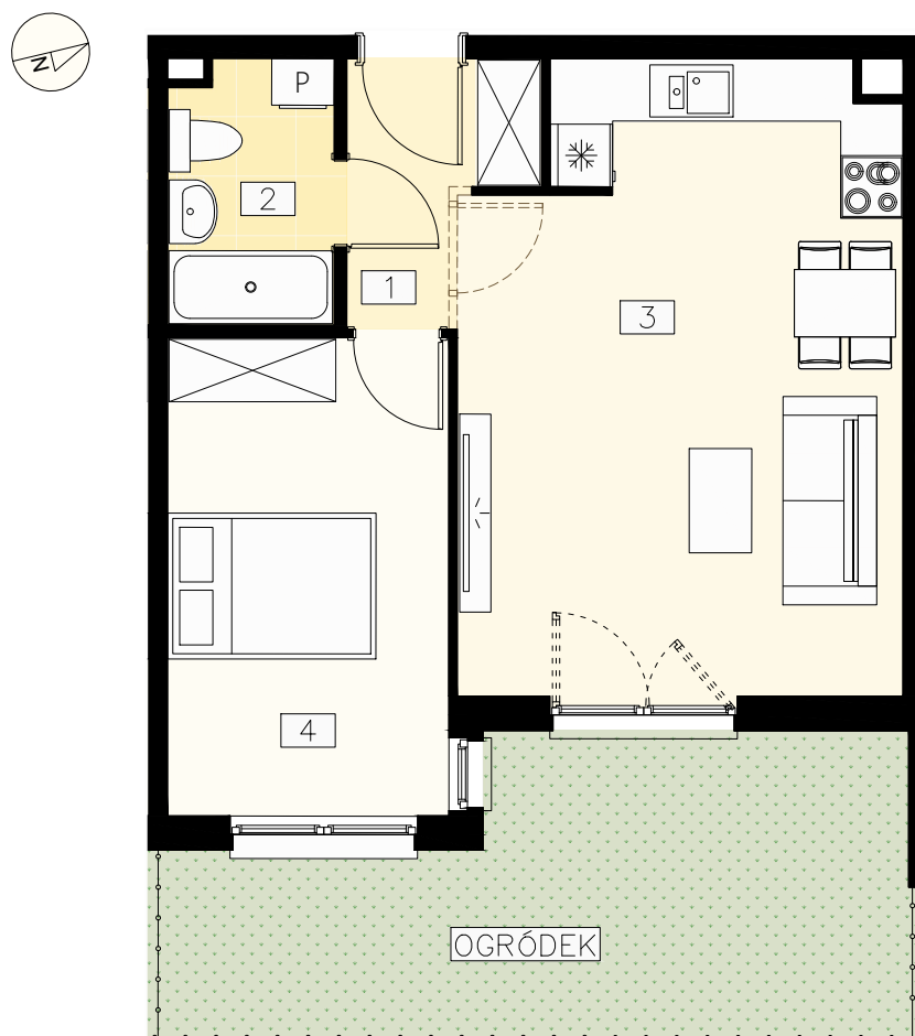
RZUT LOKALU
