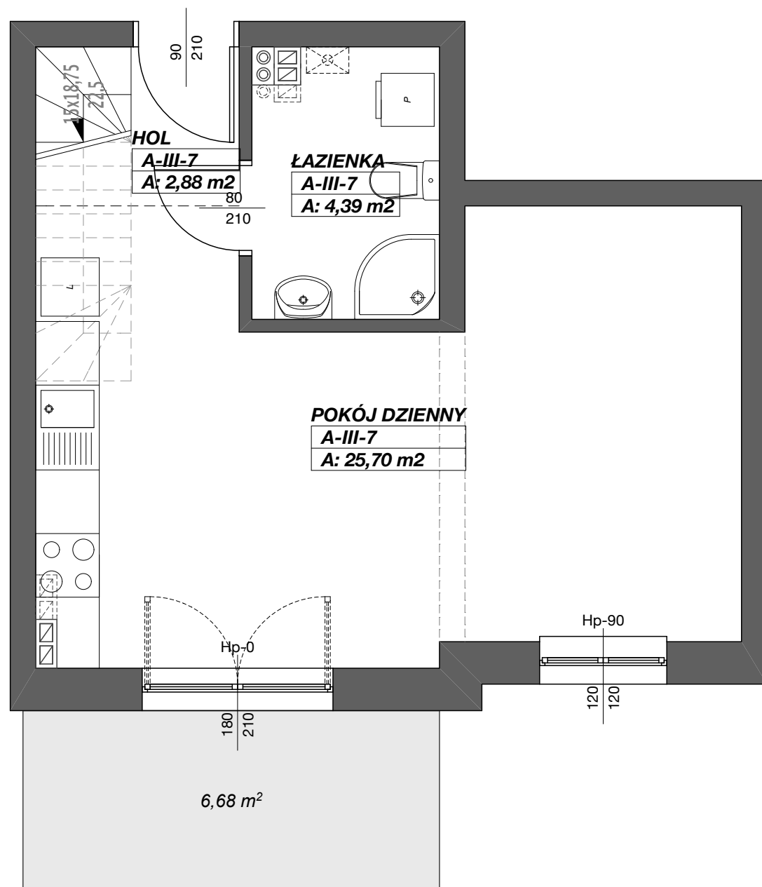
Rzut mieszkania skala 1:50
