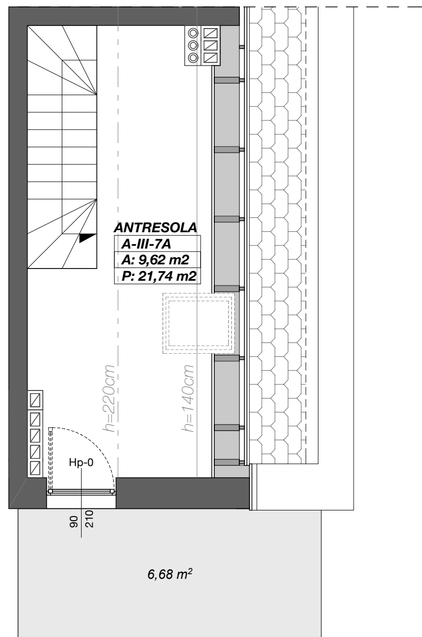
Rzut antresoli skala 1:50
