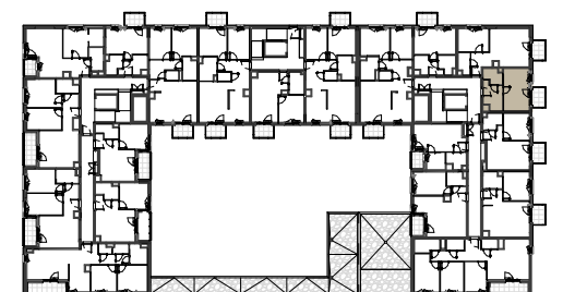
Rzut piętra 1
