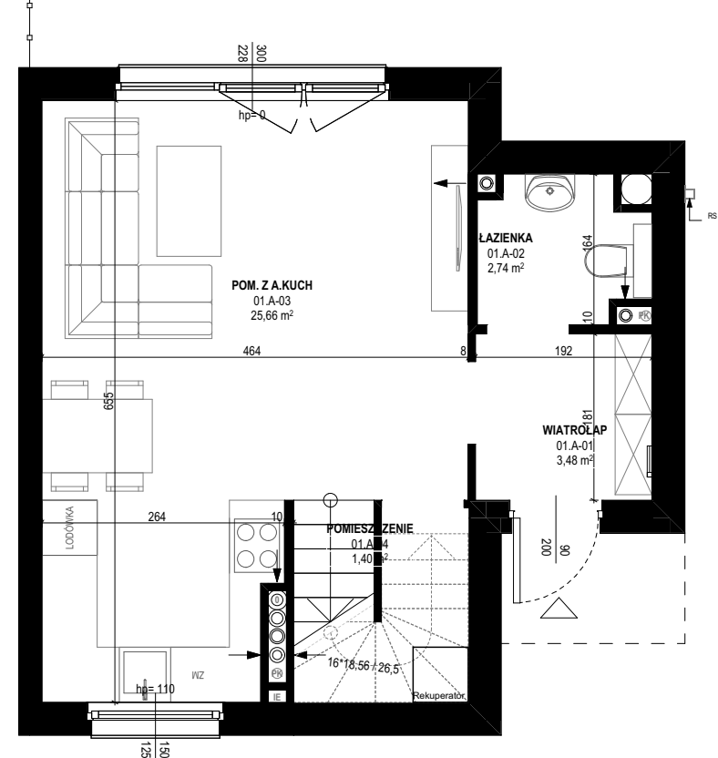
RZUT PARTERU
