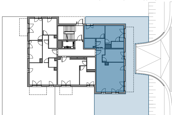
SCHEMAT LOKALU MIESZKALNEGO NA PIĘTRZE
