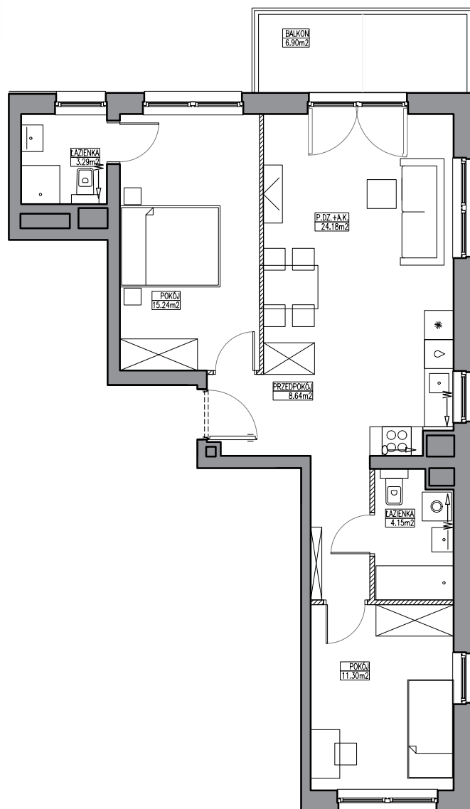
SCHEMAT LOKALU MIESZKALNEGO NA 3 PIĘTRZE
