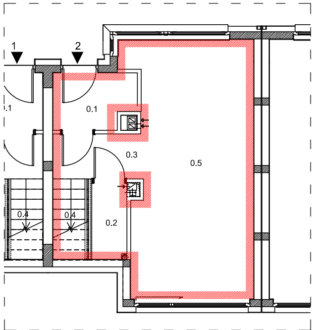
RZUT PARTERU BUDYNKU NR 11 LOKAL MIESZKALNY NR 2
