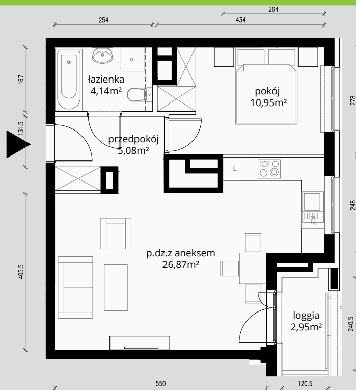
RZUT KONDYGNACJI 13 PIĘTRO
