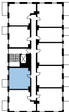
SCHEMAT LOKALU MIESZKALNEGO 4 PIĘTRZE
