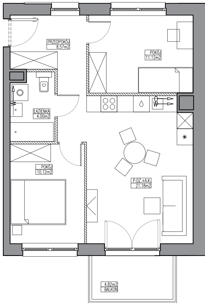
SCHEMAT LOKALU MIESZKALNEGO NA 7 PIĘTRZE
