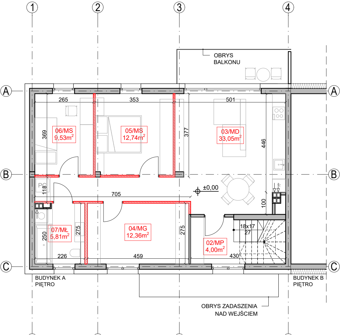
RZUT PIĘTRA
