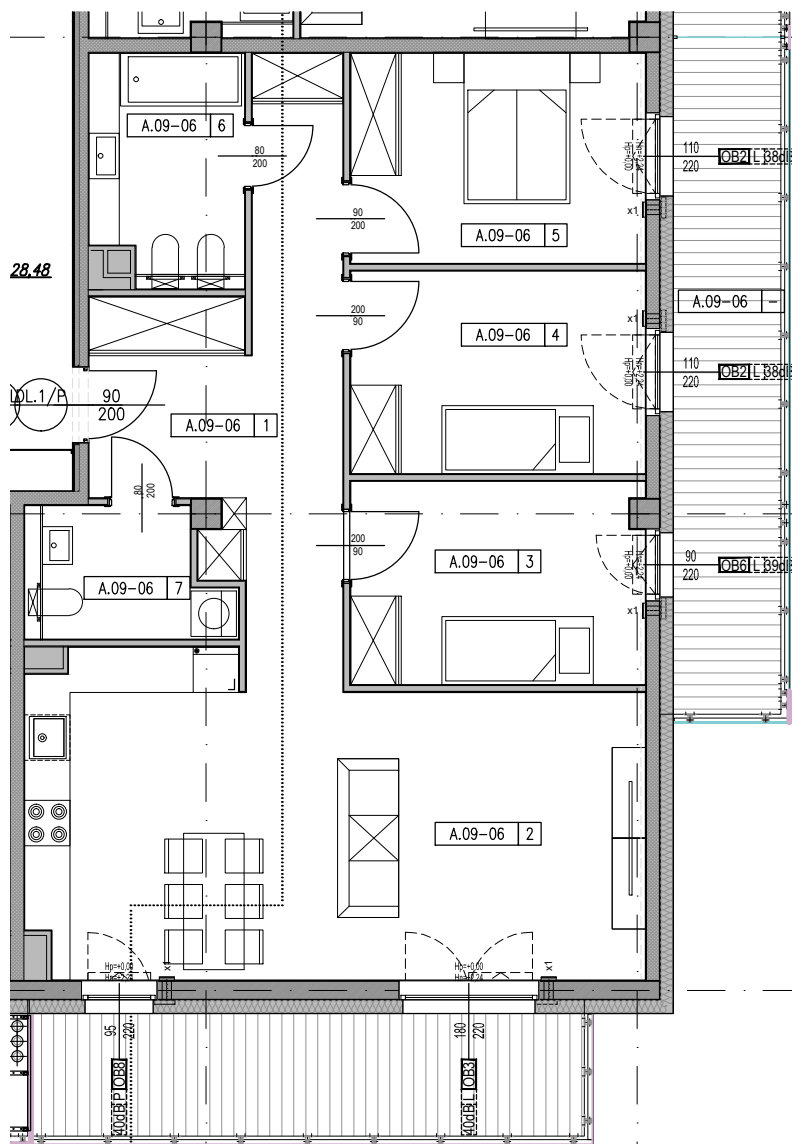
ZESTAWIENIE POWIERZCHNI - MIESZKANIE M-4P, POZIOM +9
