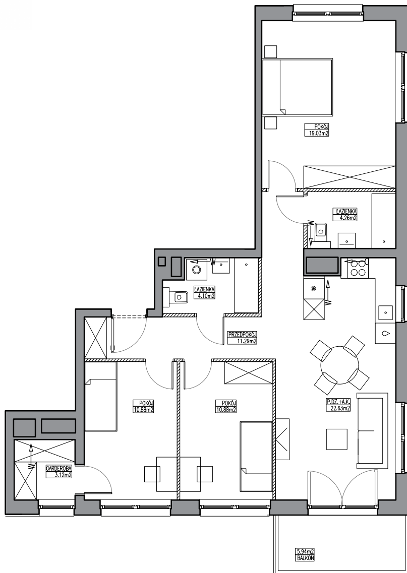
SCHEMAT LOKALU MIESZKALNEGO NA 1 PIĘTRZE
