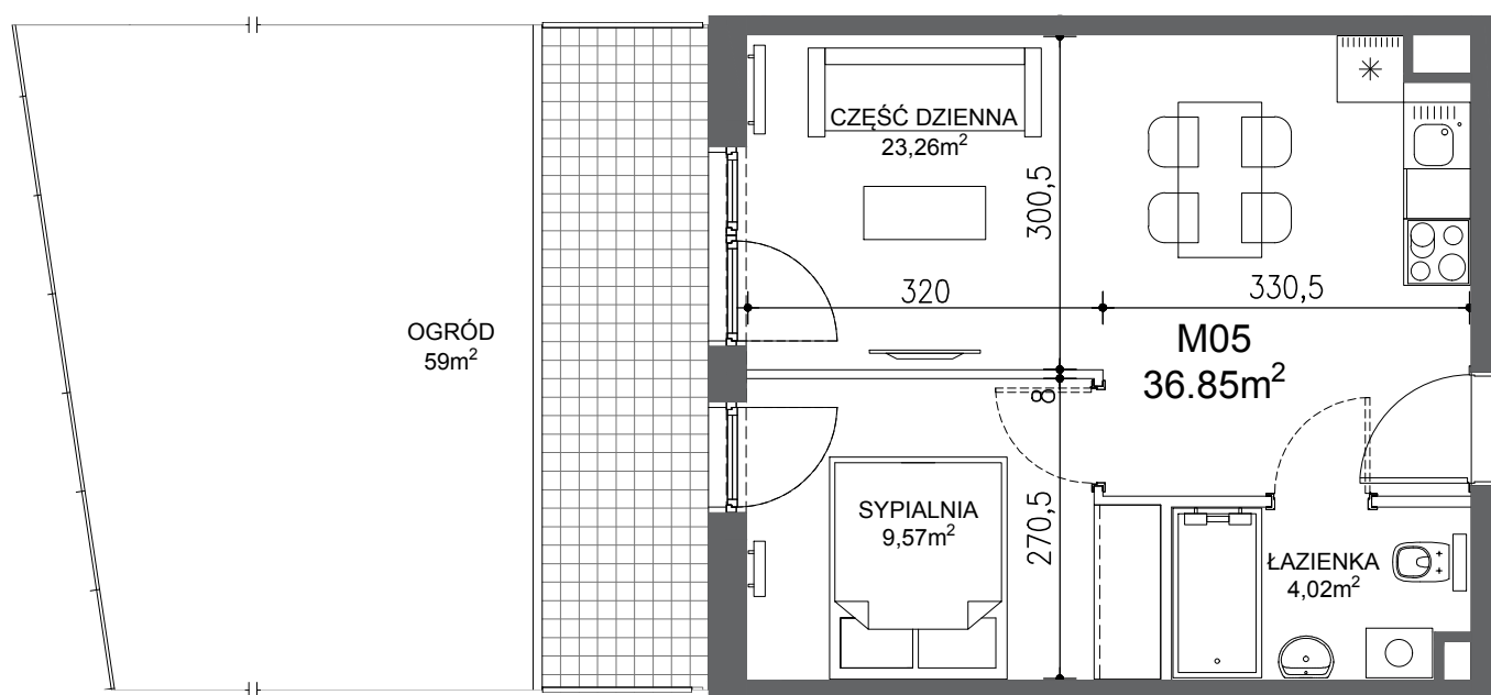
RZUT MIESZKANIA
